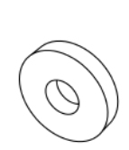
H (x3) M6, Ø:17 mm
